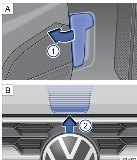
Fig. 180 [A] Palanca de desbloqueo de la tapa del compartimento del motor en la zona reposapiés del conductor. [B] Palanca de desbloqueo en la parte interior de la tapa del compartimento del motor.
