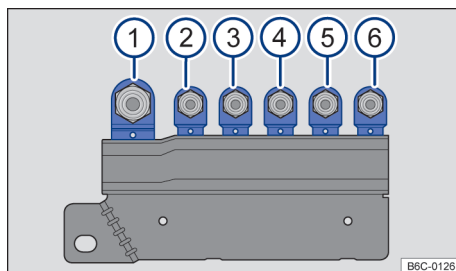
Fig. 175 En el compartimento del motor encima de la batería: disposición de los fusibles.
