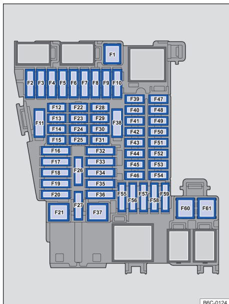
Fig. 172 En el panel de instrumentos: disposición de los fusibles.
