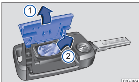
Fig. 49 Llave del vehículo: sustituir la pila.
