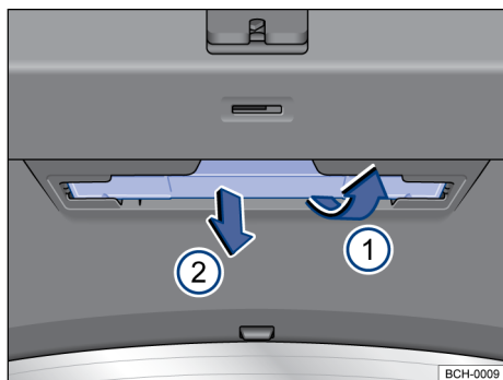
Fig. 46 En el portón trasero: soporte para el triángulo de seguridad.
