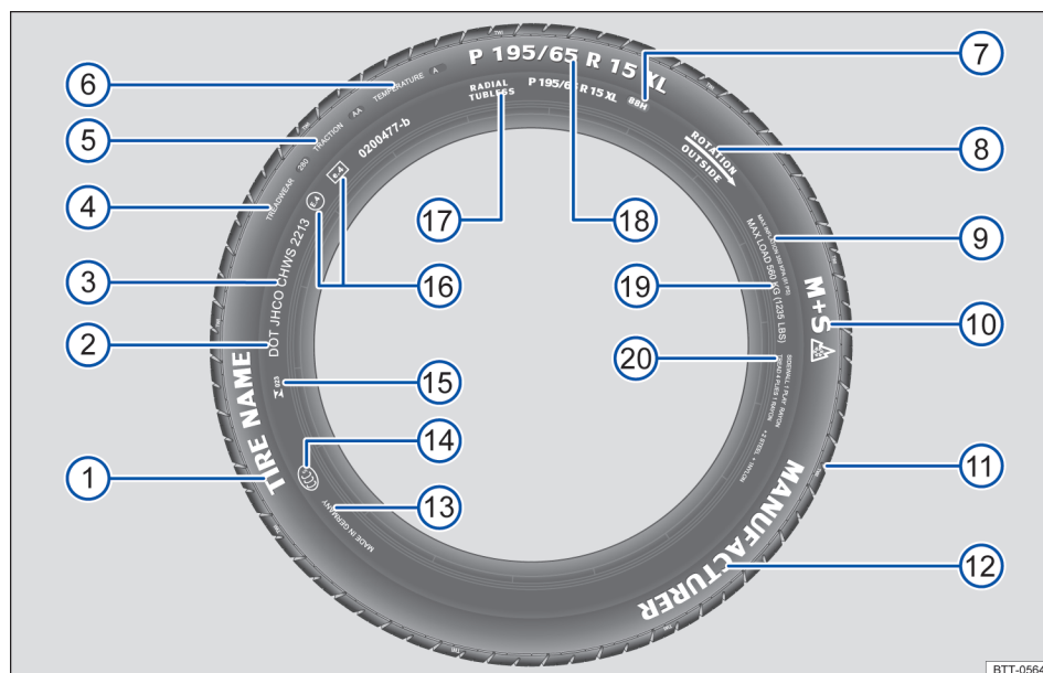
Fig. 196 Inscripción de los neumáticos internacional (ejemplo).
