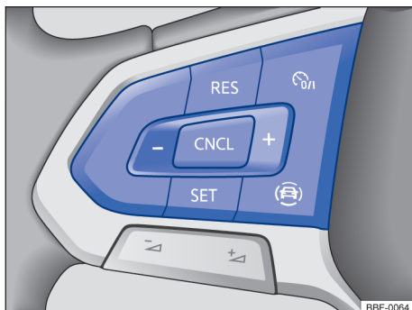
Fig. 100 Lado izquierdo del volante multifunción (variante 2): teclas para controlar el limitador de velocidad.
