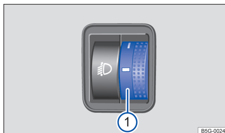
Fig. 73 Al lado del volante: ajustador de alcance de faros ①
