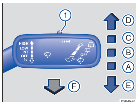
Fig. 74 A la derecha de la columna de dirección: comandar los limpiavaparabrisas.
