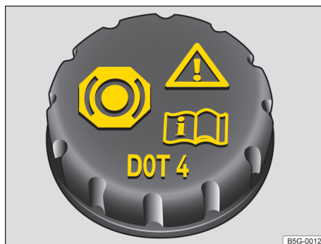
Fig. 188 En el compartimento del motor: tapón de cierre del depósito del líquido de frenos.
