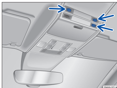
Fig. 57 En la consola del techo: sensores de vigilancia del habitáculo (flechas).
