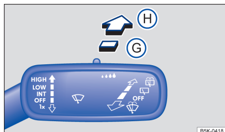
Fig. 75 A la derecha de la columna de dirección: comandar el limpiavaluneta.
