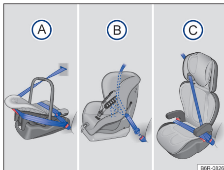
Fig. 39 Las ilustraciones A, B y C muestran la fijación del sistema de retención infantil solo con el cinturón de seguridad del vehículo.
