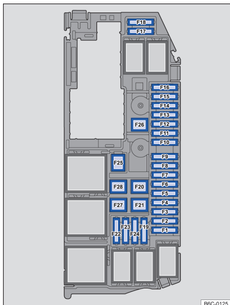
Fig. 174 En el compartimento del motor: disposición de los fusibles.
