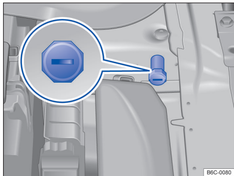
Fig. 178 En el compartimento del motor: punto de ayuda de arranque (punto de conexión a tierra).
