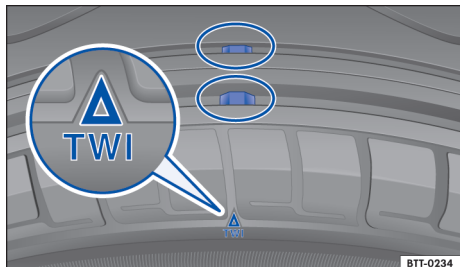
Fig. 194 Perfil del neumático: indicadores de desgaste.
