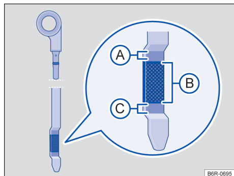
Fig. 184 Varilla de medición del aceite con marca de nivel de aceite del motor.
