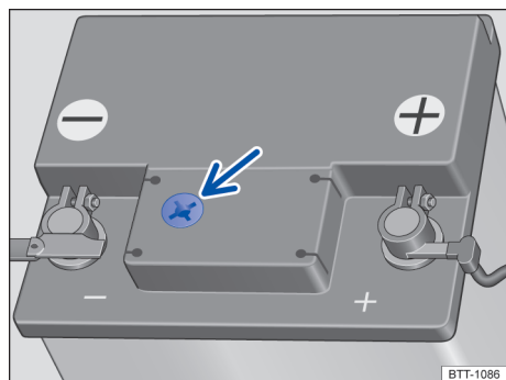
Fig. 189 En el compartimento del motor: ejemplo de posición del visor en el lado superior de la batería del vehículo.
