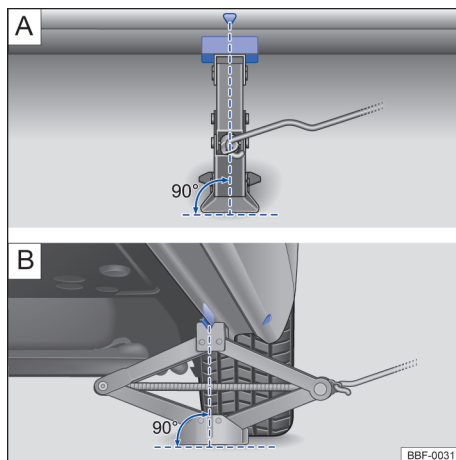
Fig. 199 Puntos de apoyo del gato y gato posicionado atrás en el lado izquierdo trasero del vehículo.
