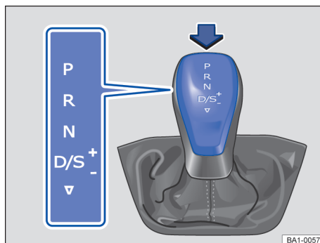
Fig. 93 Palanca selectora de la transmisión automática con tecla de bloqueo (flecha).
